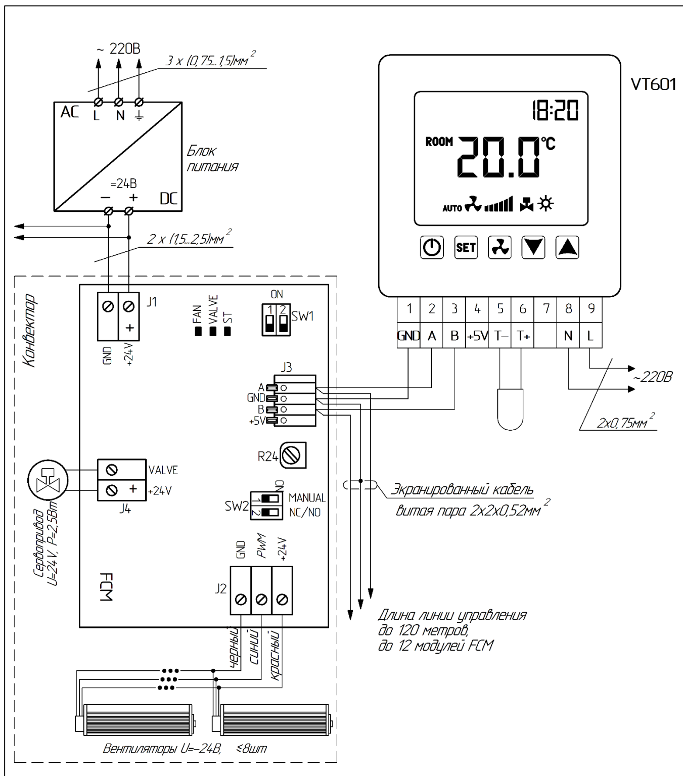
Схема соединений для Бриз В 24В (вентиляторы 24В постоянного тока с ШИМ-управлением).
