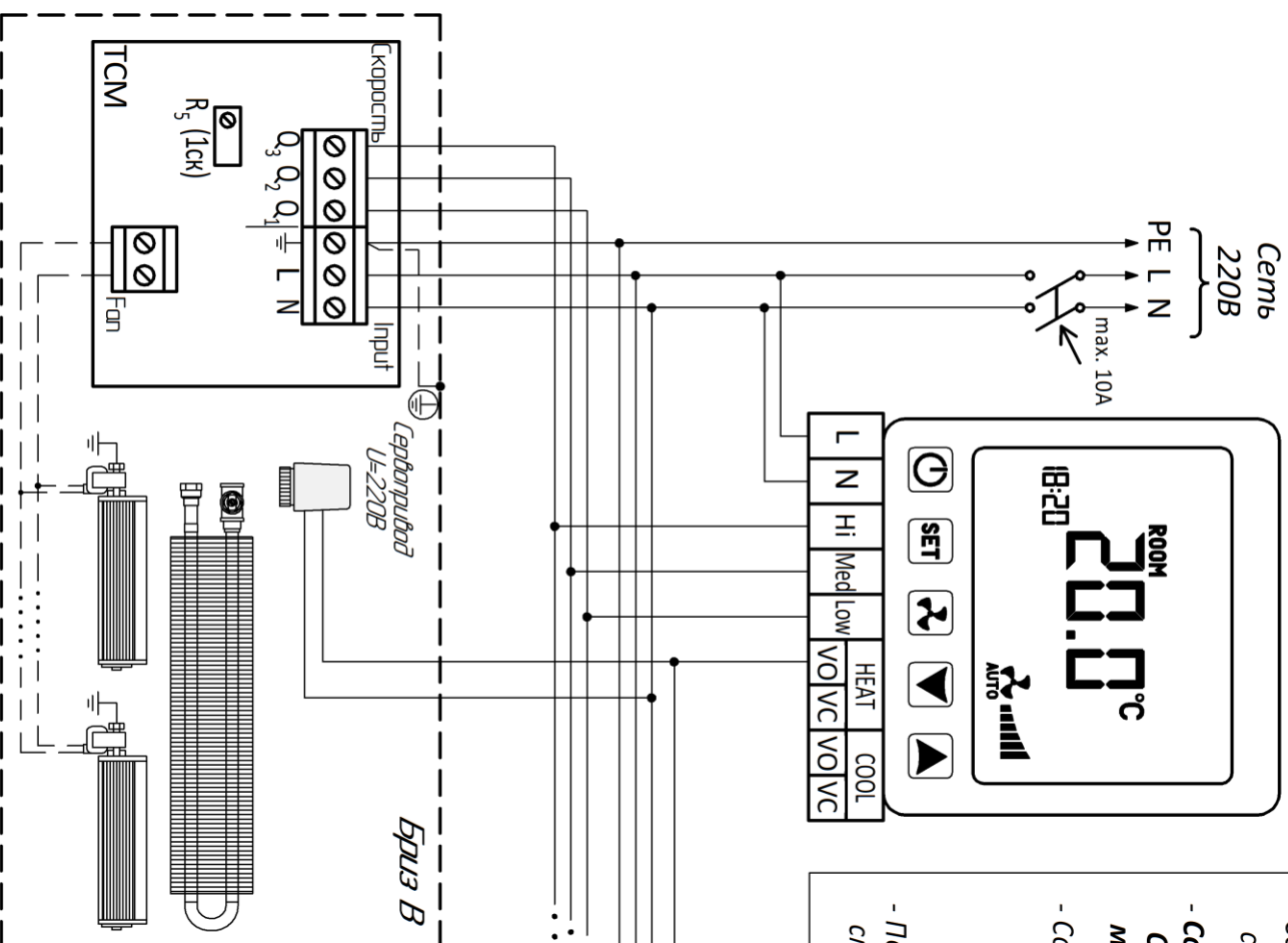
Схема соединений модуля TCM и термостата "VT301" для трехступенчатого управления вентиляторами U = 220В конвекторов "Брыз В"
